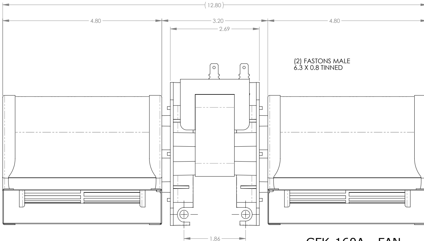
GFK-160A - FAN 100MM-V-P
