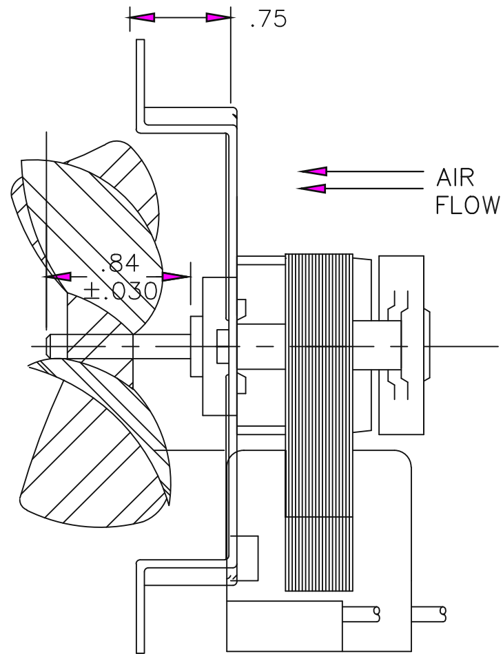
FK1 - FK2 - FK18 - 1CFMS FAN 4" Blade Fan
