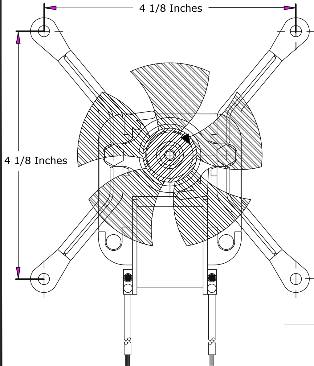
BK3 - FAN 4" Blade Fan
